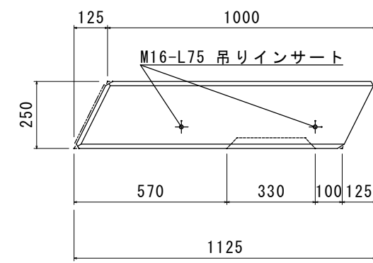
B矢視立面図
