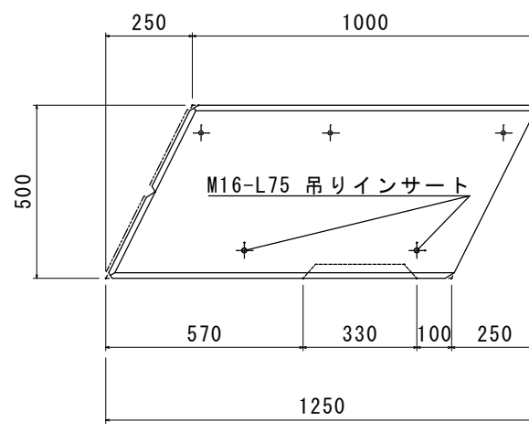
B矢視立面図
