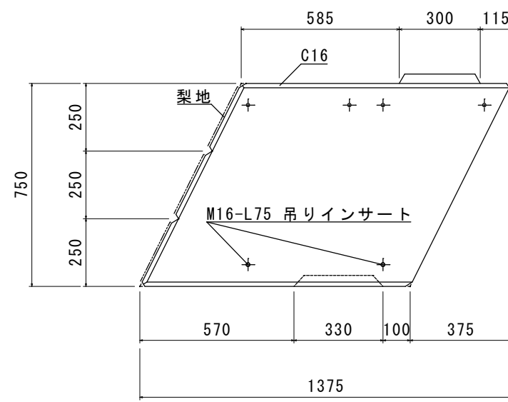
B矢視立面図
