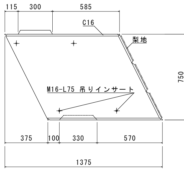
B矢視立面図
