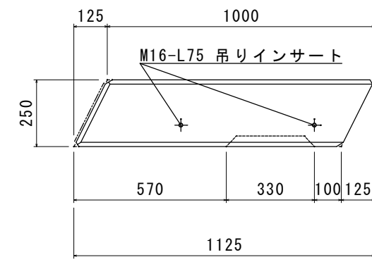
A矢視立面図
