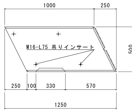
B矢視立面図
