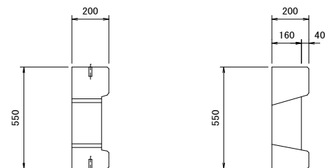
B-B
