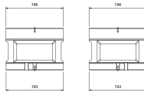
半丁ブロック基礎
