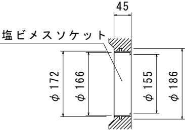
A 部詳細図(埋込み部) ※S=1/10
