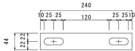
連結プレート t=3.2mm
