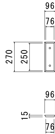
連結部詳細図
