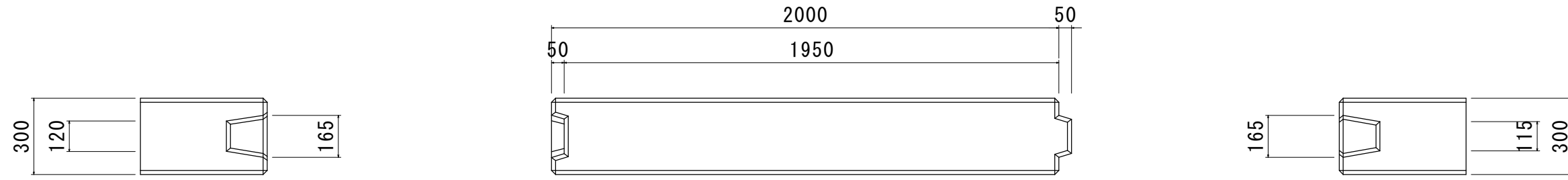
側面図
