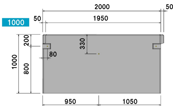
連結部詳細図
