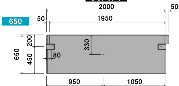
側面図
