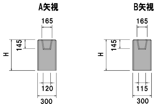
正面図
