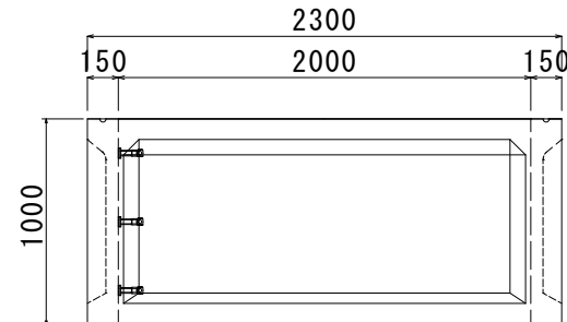
側面図
