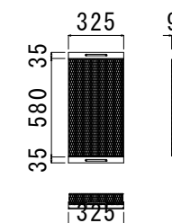
OKザールフィルター (雨水協認定品)
