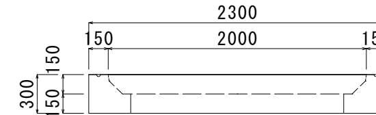
側面図
