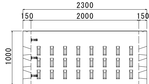
側面図
