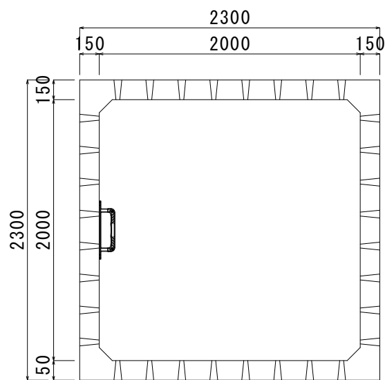
平面図
