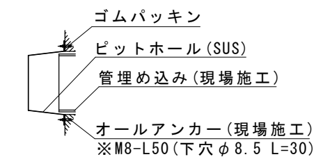
ピットホール取付詳細図
