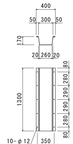
ピットホール (標準) (SUS製 t=0.8mm)
