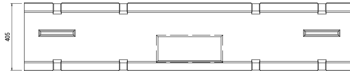
底面図 (管理孔)
