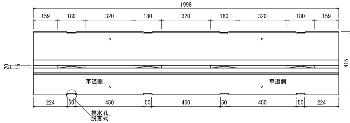
側面図(標準)
