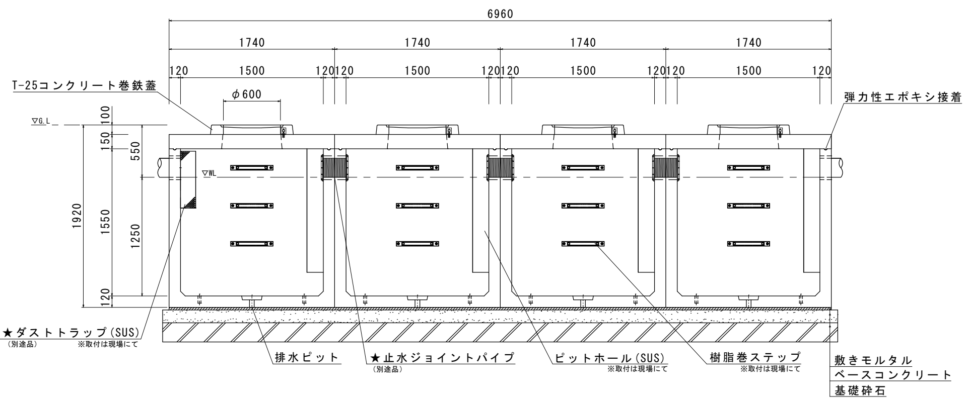
正面断面図
