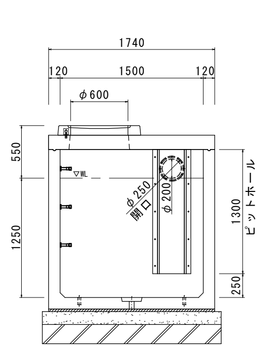
A-A断面図
